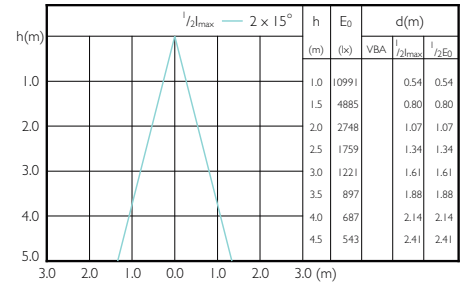
LEDspot PAR30L E27 5700K 30D
